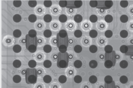
▲ BGA: 90kV 100μA
