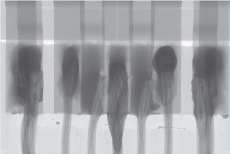
▲ ハンダ接合：90kV 100μA
